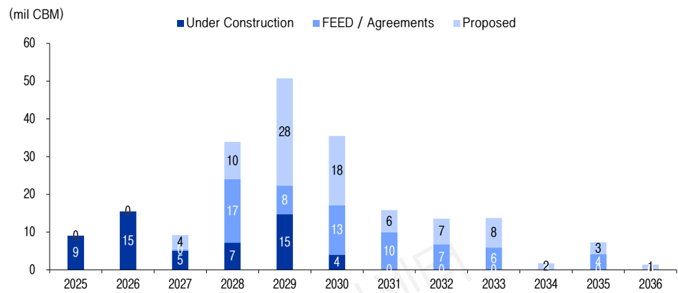
그림37 글로벌 LNG 액화플랜트 프로젝트 신규 추진에 따른 LNGC 필요 선복량
