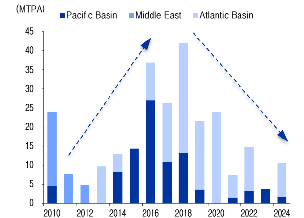
그림14 연간 지역별 LNG Liquefaction Facility 신설 Capa
