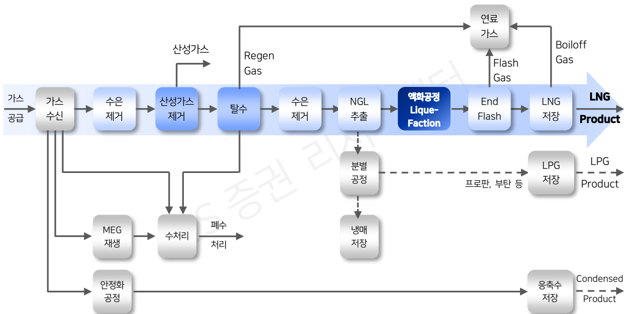
그림22 FLNG 공정 모식도
