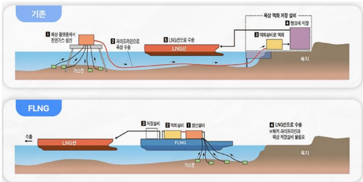
그림21 FLNG: 해저 파이프라인과 육상 저장설비 불필요
