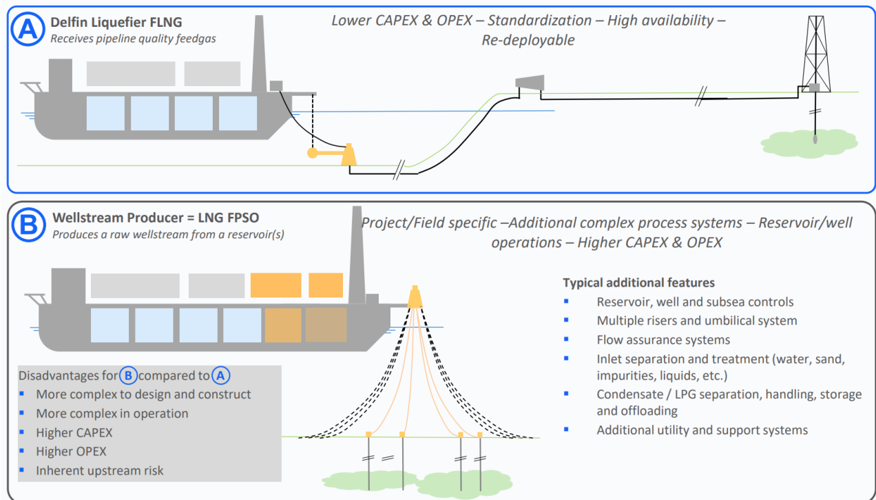
그림23 Delfin Liquefier: 전처리 단계를 마친 '파이프라인 퀄리티' 가스만을 처리. 구조 단순화. 설계 표준화. 비용 절감 효과
