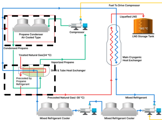
그림99 LNG 액화 공정에서 Air Cooler 역할
